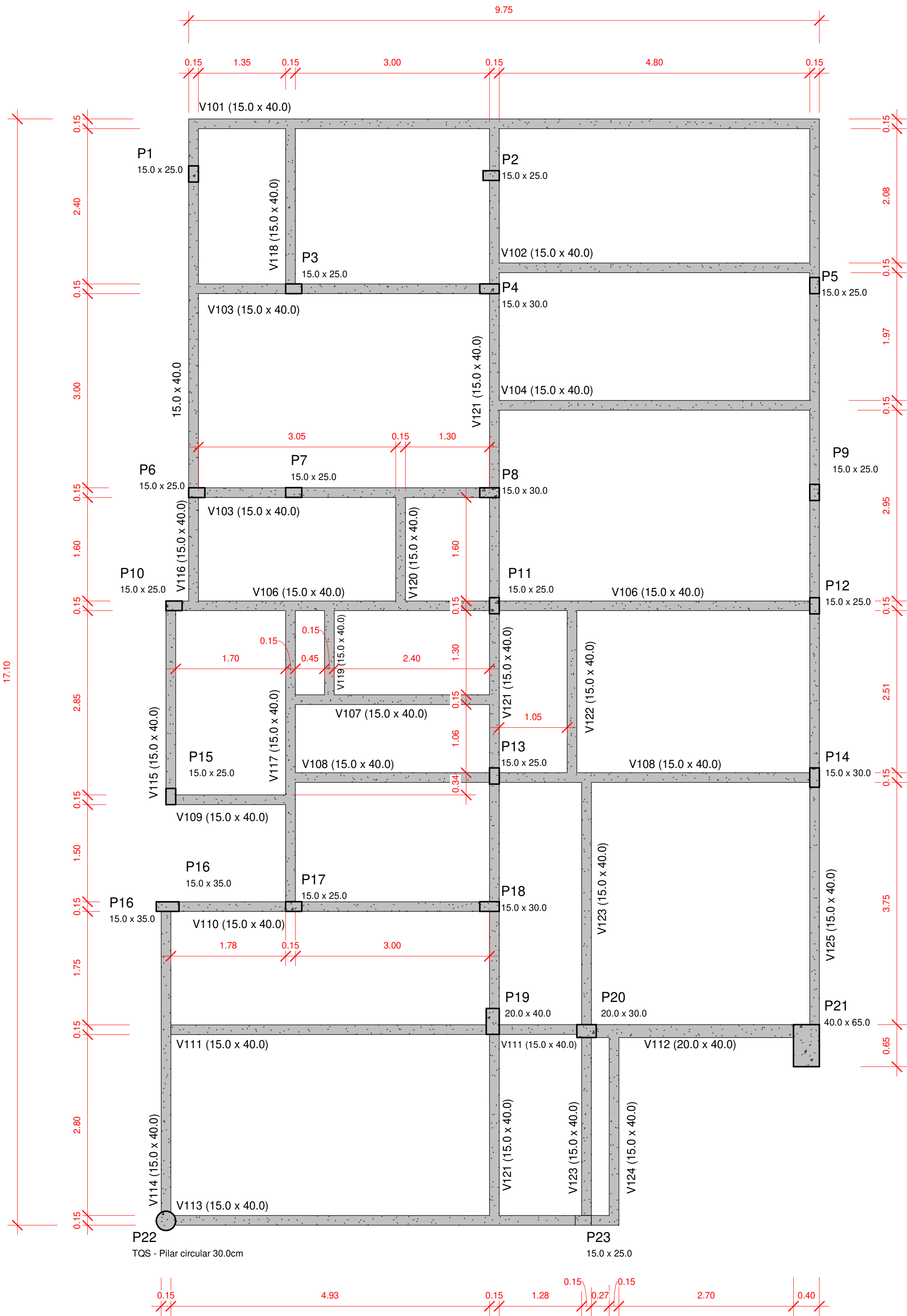
PLANTA DE FORMA - BALDRAME 1 : 50
