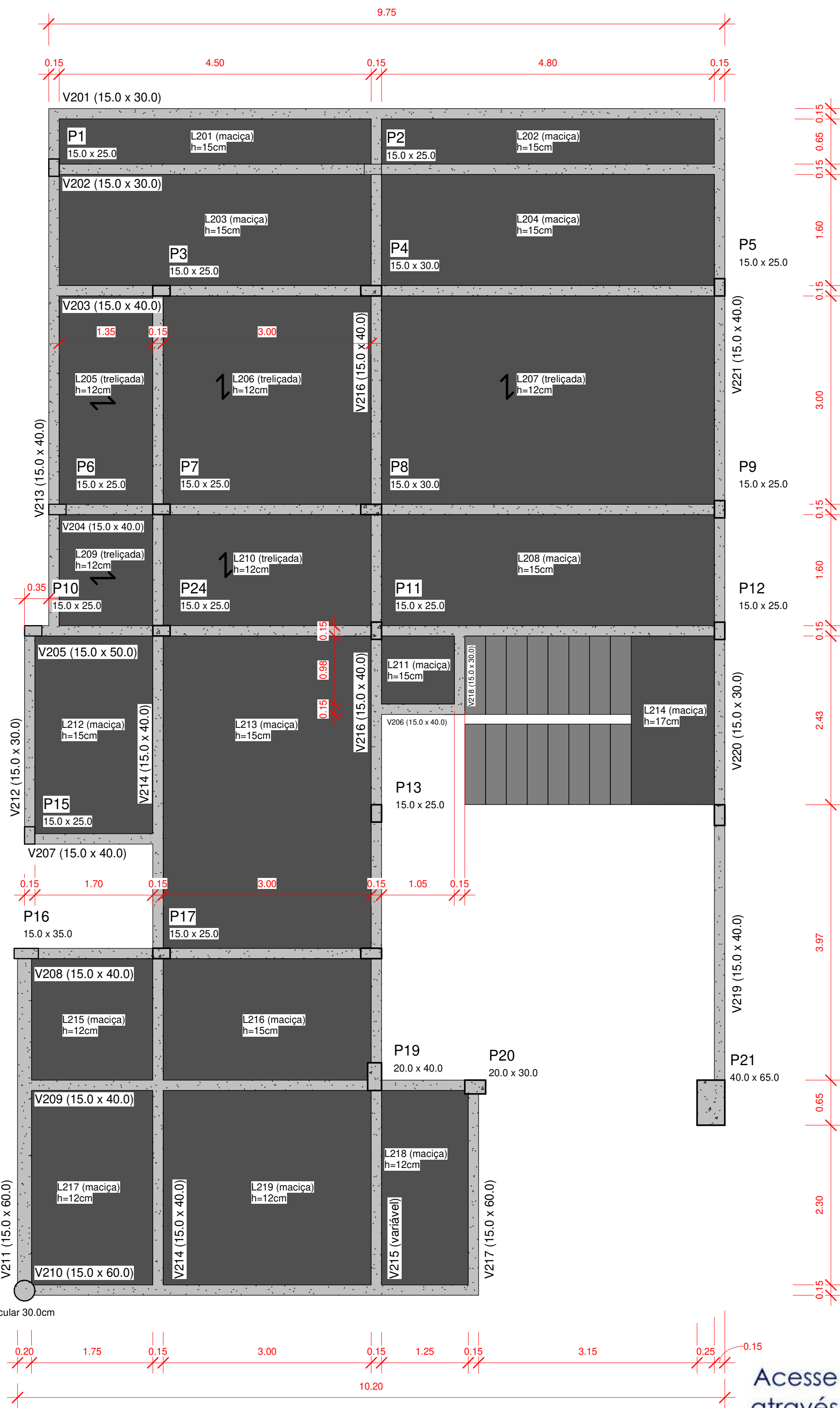
PLANTA DE FORMA - 1º PAVIMENTO 1 : 50
